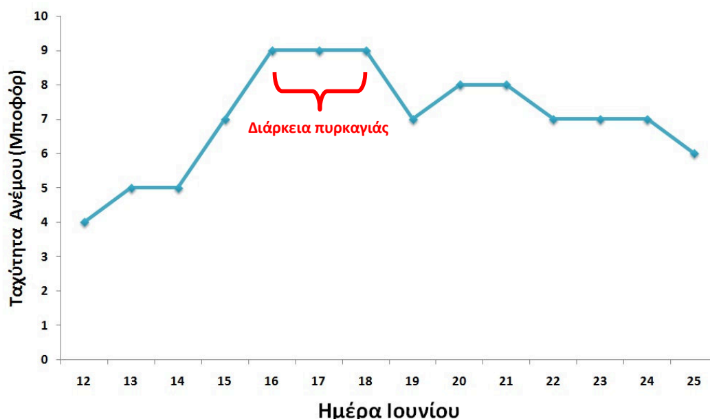
Σχήμα 1: Μέγιστη ημερήσια ταχύτητα ανέμου (μποφόρ) στα μέσα του μήνα Ιούνι, οπότε και εκδηλώθηκε η πυρκαγιά στη Λαυρεωτική. Πηγή δεδομένων: Εθνικό Αστεροσκοπείο Αθηνών, μετεωρολογικός σταθμός Λαυρίου - http://penteli.meteo.gr/stations/lavrio/ .
