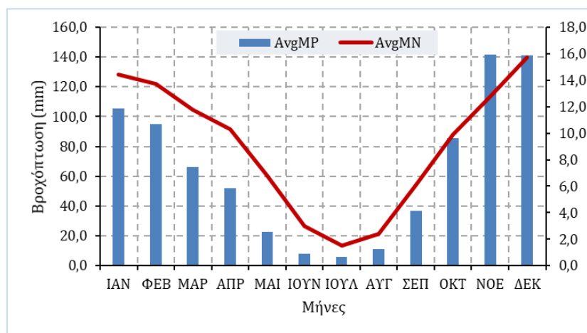
Εικόνα 5.5: Γράφημα υετού για την περιοχή Ανατολικής Μάνης. (Πηγή: EMY)
