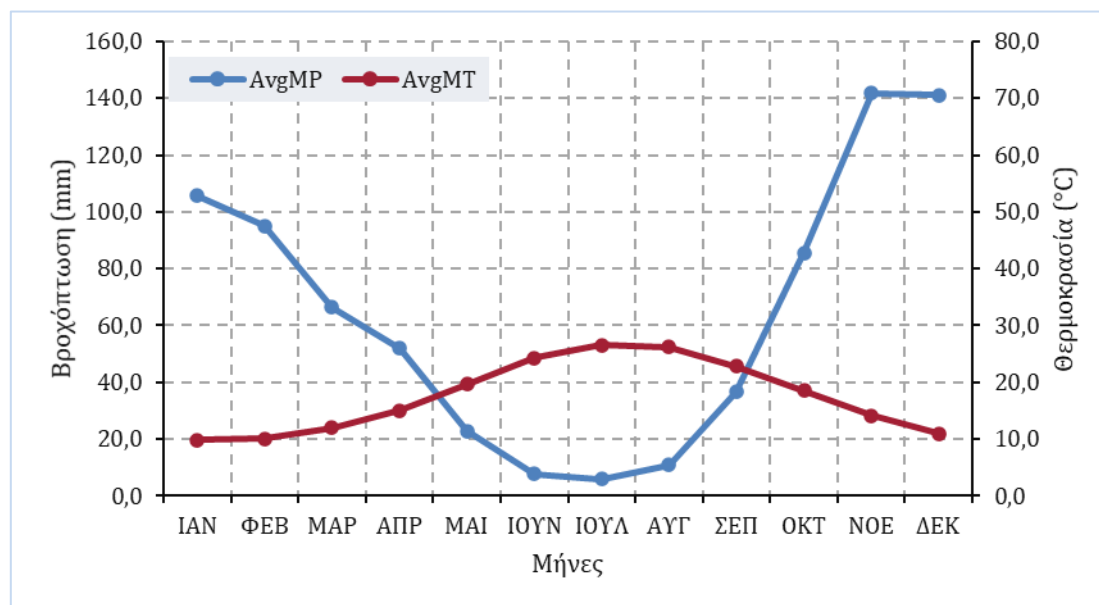
Εικόνα 5.8: Ομβροθερμικό διάγραμμα για την περιοχή Ανατολικής Μάνης. (Πηγή: EMY)
