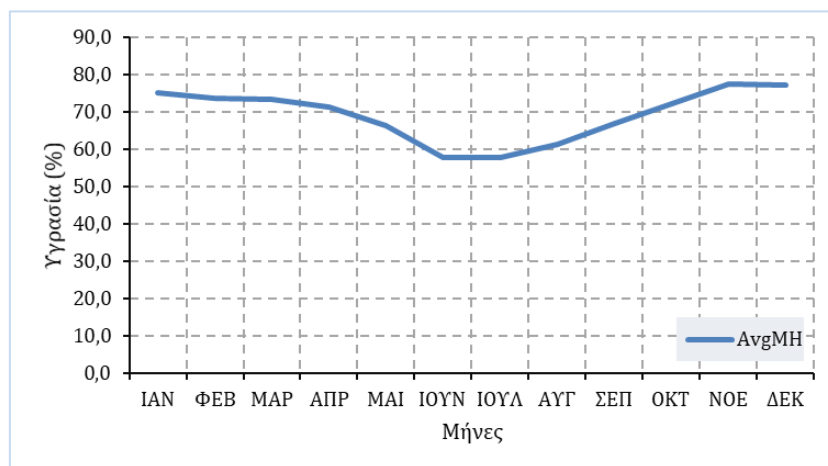
Εικόνα 5.4: Γράφημα μέσης μηνιαίας υγρασίας για την περιοχή Ανατολικής Μάνης. (Πηγή: EMY)
