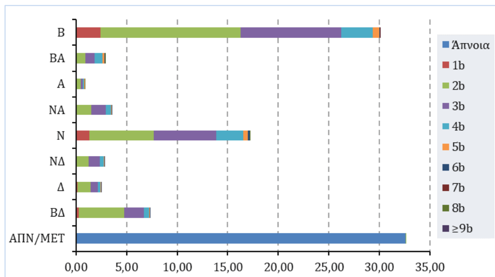
Εικόνα 5.7: Γράφημα ετήσιων συχνοτήτων ανέμου για την περιοχή Ανατολικής Μάνης. (Πηγή: EMY)
