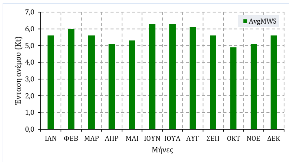
Εικόνα 5.6: Γράφημα ανέμου για την περιοχή Ανατολικής Μάνης. (Πηγή: EMY)
