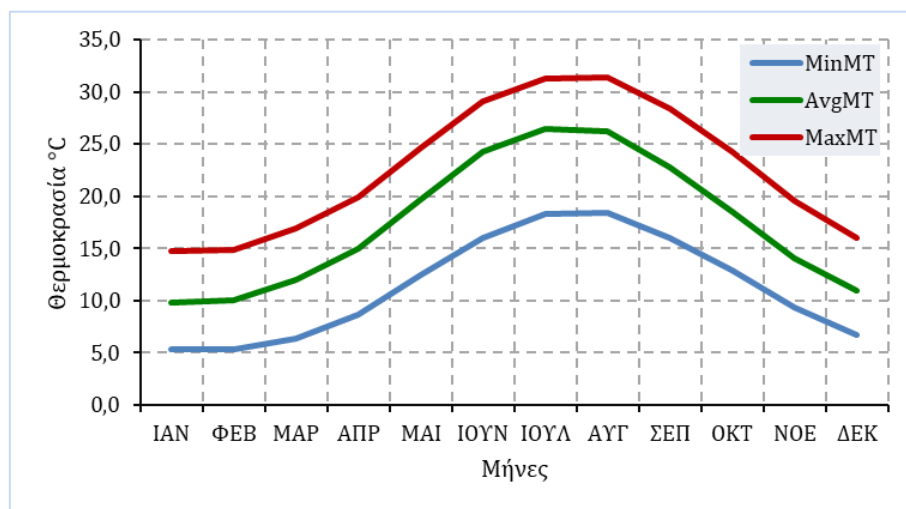
Εικόνα 5.3: Γράφημα θερμοκρασίας για την περιοχή Ανατολικής Μάνης. (Πηγή: EMY)
